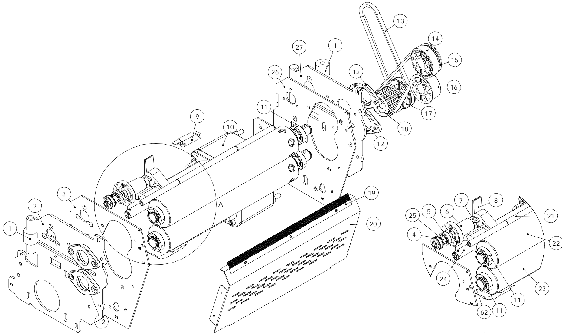
상세 A 배율 1:2
